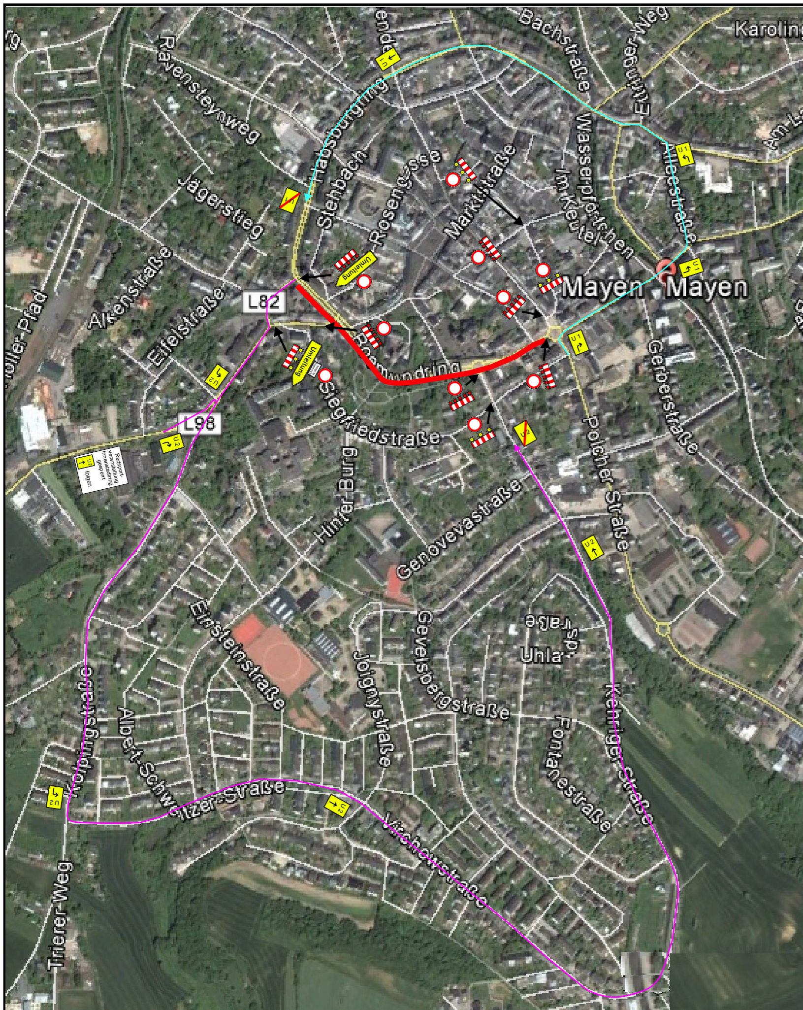
Detailplan Umleitung
